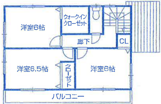
2階平面図
